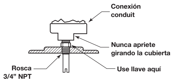
Figura 3 Montaje Vertical
