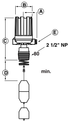
Modelle A10/A15/B10/B15 Gewindeanschluss
