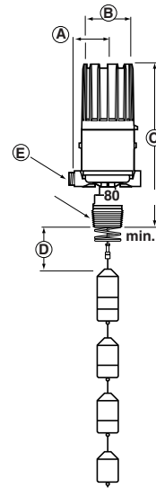
Modelle C10/C15 Gewindeanschluss
